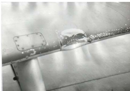
5. ábra A bal felszárnny belépő éle
