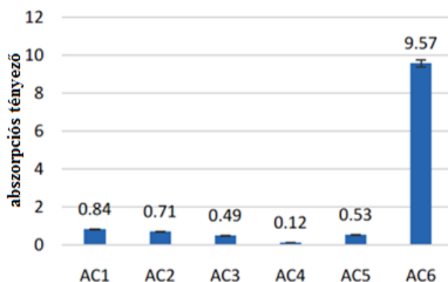
6. ábra Az aktív szenek \epsilon'' abszorpciós tényezői [7]
