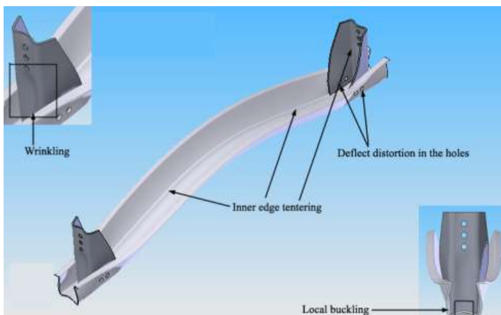
10. ábra – U profil helyenkénti deformációi, károsodási zónái; az angol megnevezések magyar megfelelői: wrinkling – gyűrődés, tenting – feszítő nyúlás, local buckling – helyi kihajlás, deflect distortion in the holes – szeges furat eltorzulása
