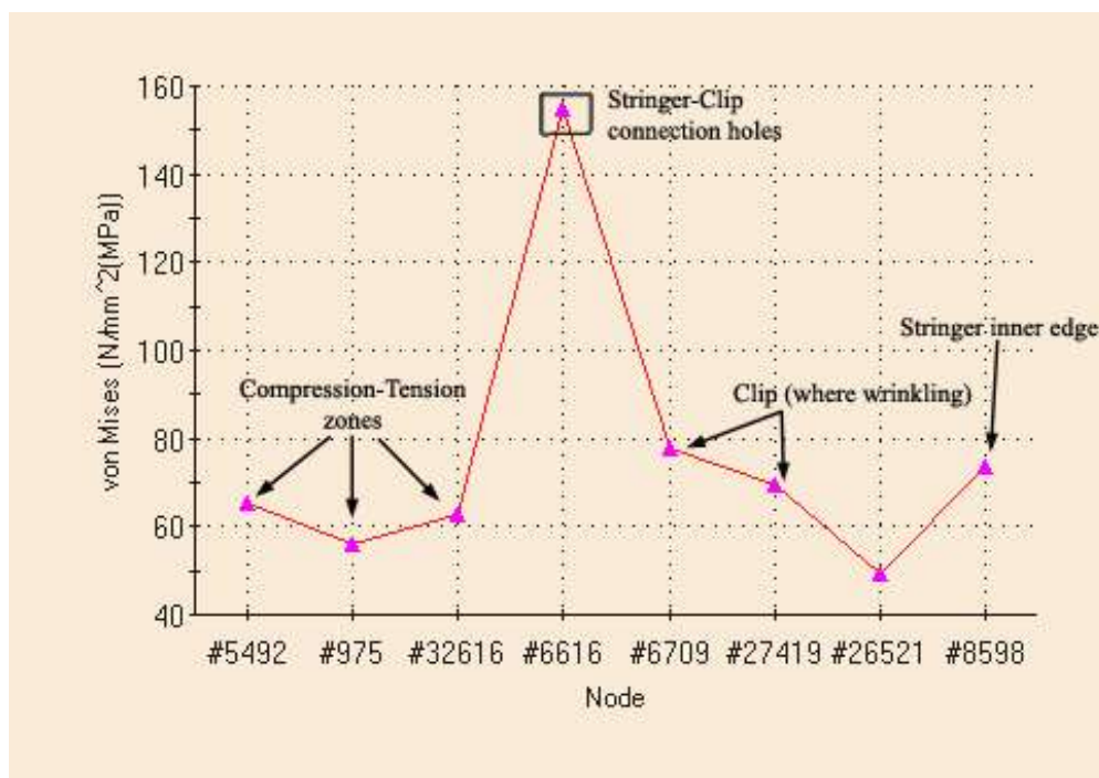
12. ábra – Feszültségek lokális értékei, az angol megnevezések magyar megfelelője: Compression-tension zones – nyomási-húzási zónák, stringer-clip connection holes – hossztartó-pánt kapcsolatok furatai, clip (where wrinkling) – pánt ahol a gyűrődés ébred, stringer inner edge – hossztartó belső éle
