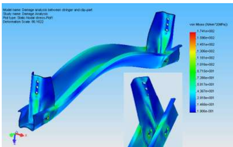
11. ábra – Feszültség eloszlási térkép
