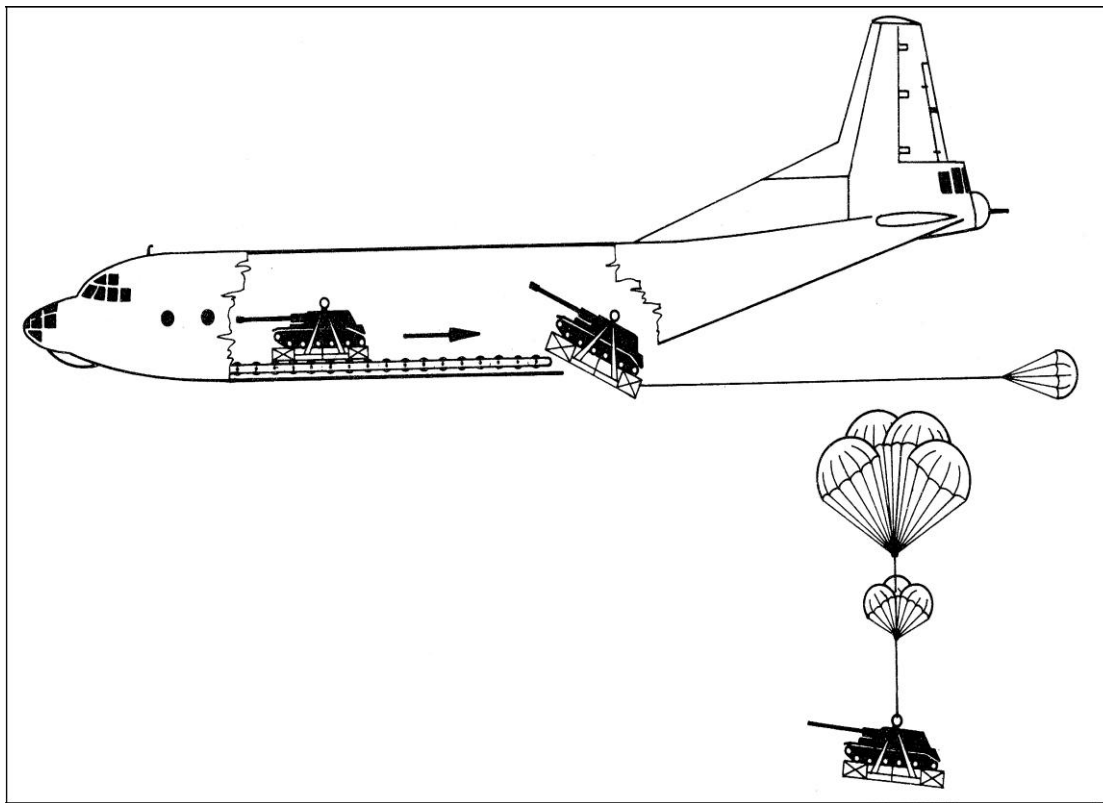
5. ábra. Légideszant-harcjármű deszantolása terepre tehertejőernyő-rendszerrel
