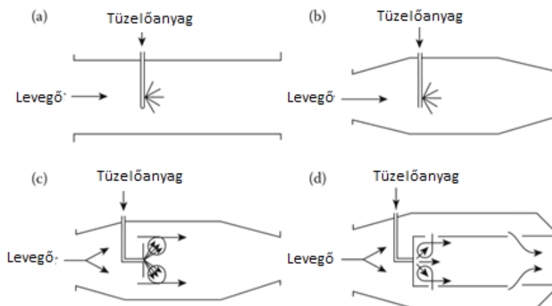
15. ábra: Hagyományos égőtér konfiguráció származtatása [25]
