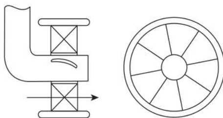
19. ábra: Axiális lapátos örvénykeltő [25]
