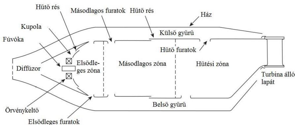
18. ábra: Az égőtér fő szekciói [20] [25]
