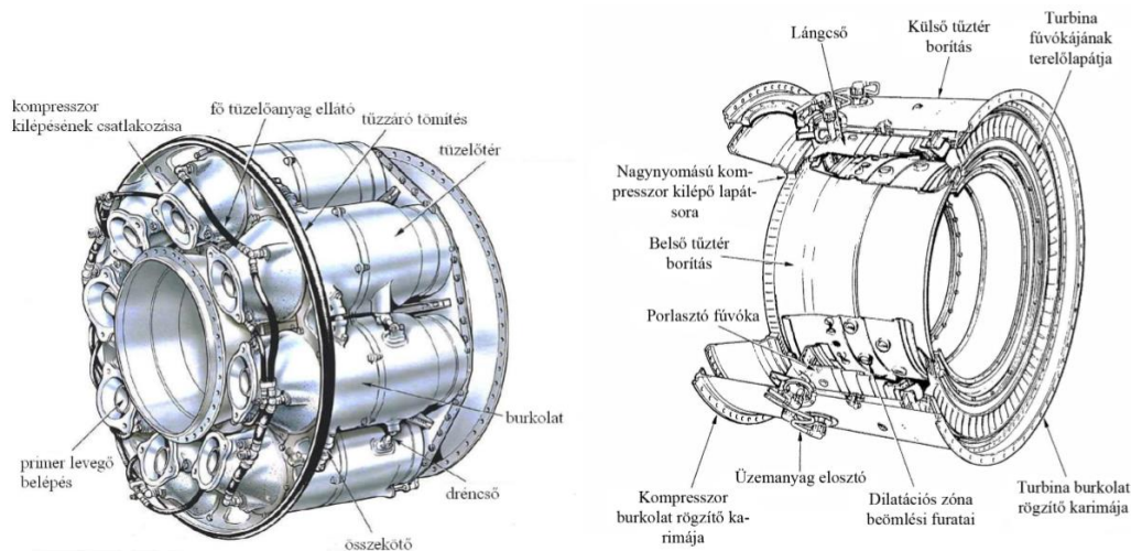
16. ábra: Csöves (balra) és gyűrűs (jobbra) égőterek [26]
