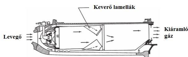
4. ábra: BMW 003-as hajtómű égőterének sematikus rajza [20]
