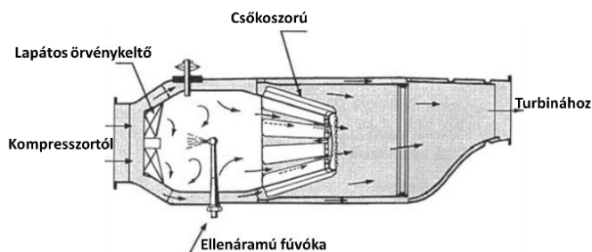
2. ábra: Jumo 004-es hajtómű égőterének sematikus rajza [20]
