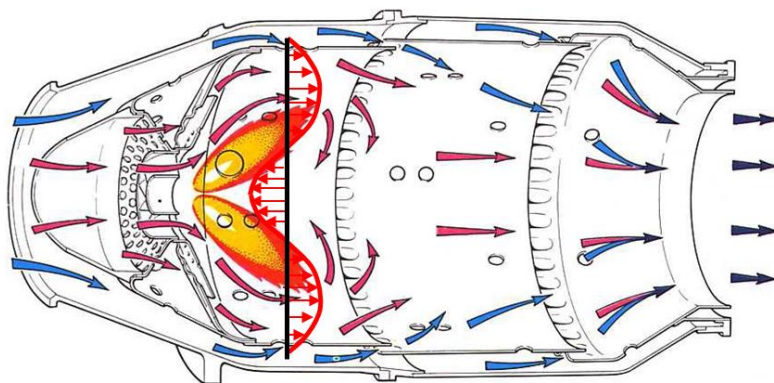
20. ábra: Áramlások az égőtérben [22] [26]
