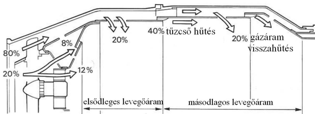
21. ábra: A tűzcsőbe bejutó levegőmennyiség eloszlása [23] [26]
