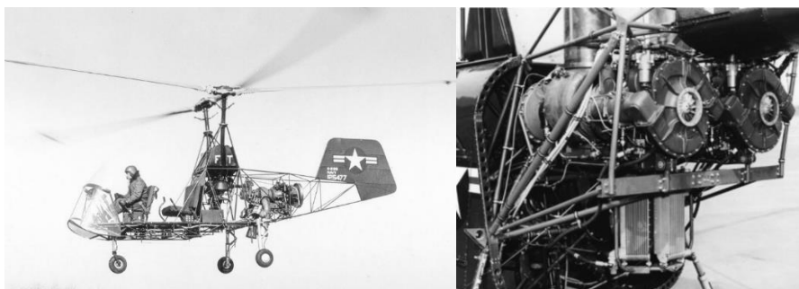
13. ábra: K-225 típusú szinkropter [16] és Boeing 502-2-es gázturbinás hajtómű [17]
