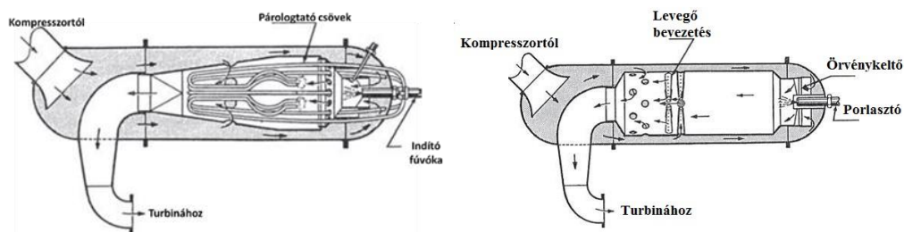
6. ábra: A "Whittle Unit" párolgató és porlasztós égőterének sematikus rajza [20]
