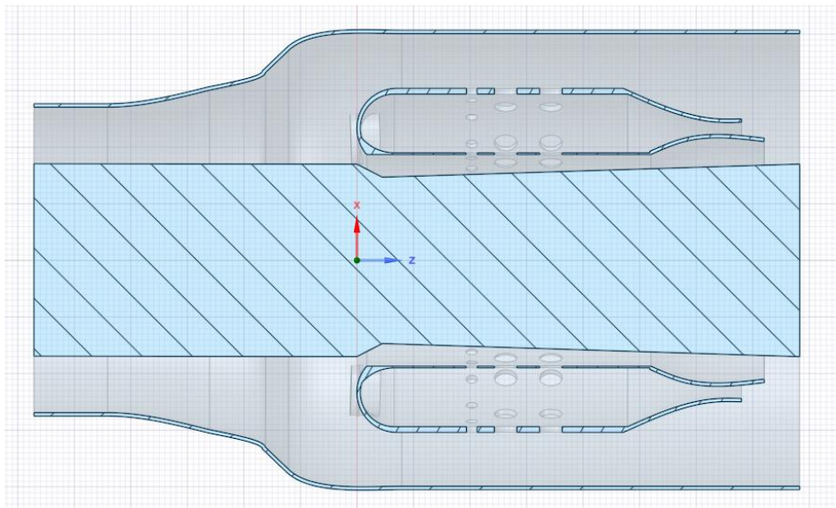
31. ábra: Az égőtér modelljének keresztmetszete ANSYS SpaceClaim környezetben (saját kép)
