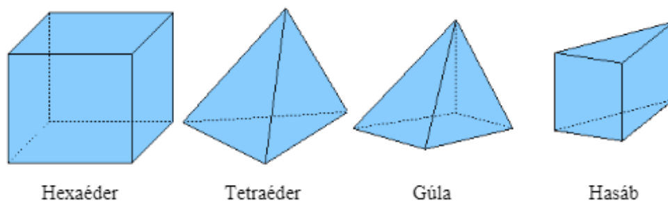
32. ábra: Az alapvető háromdimenziós hálóelemek [41]
