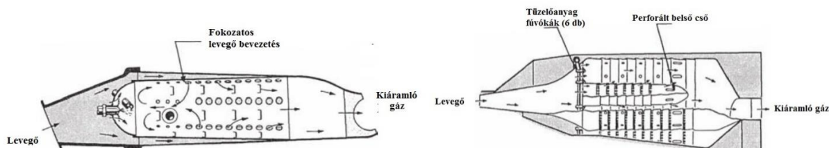
11. ábra: J33 és J57 hajtóművek égőtérének sematikus rajza [20]
