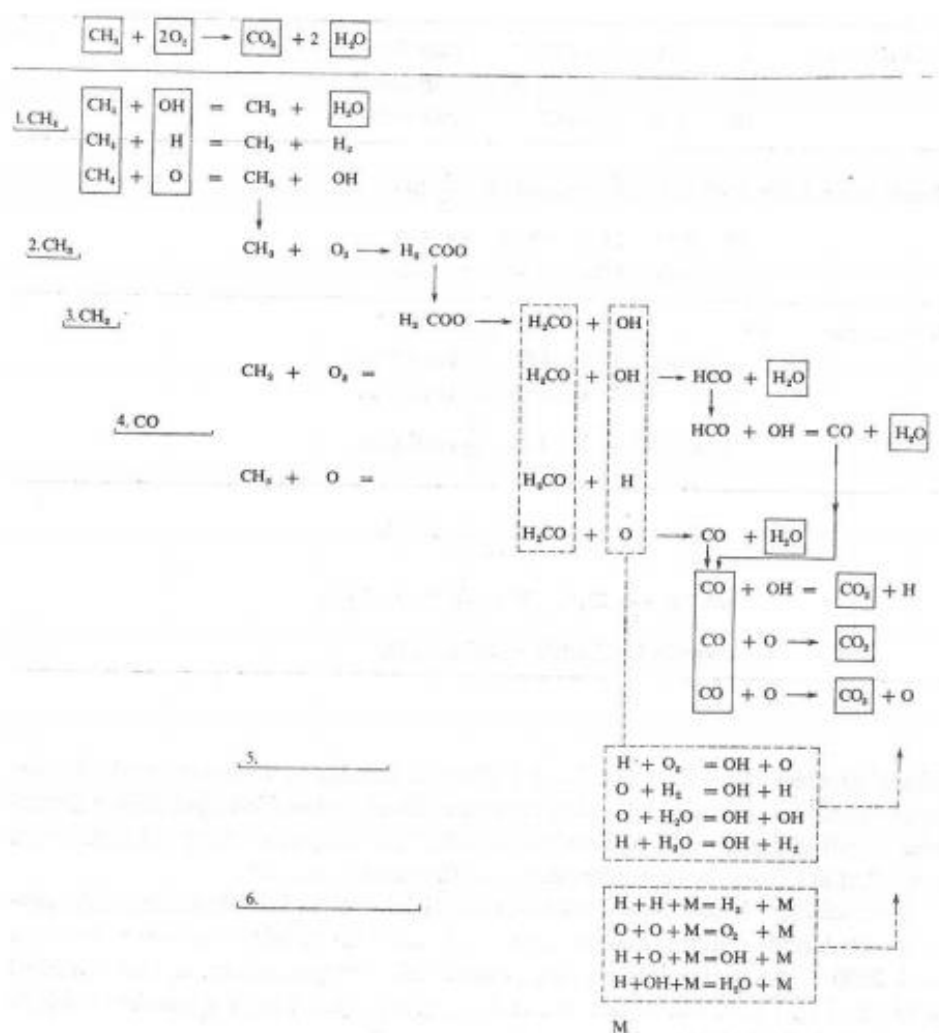
22. ábra: Metán égésének részfolyamatai [9]
