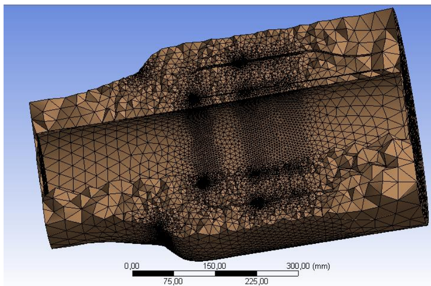
33. ábra: Égőtér tetraéderes hálós metszete egy szimmetriatengely mentén (saját kép)
