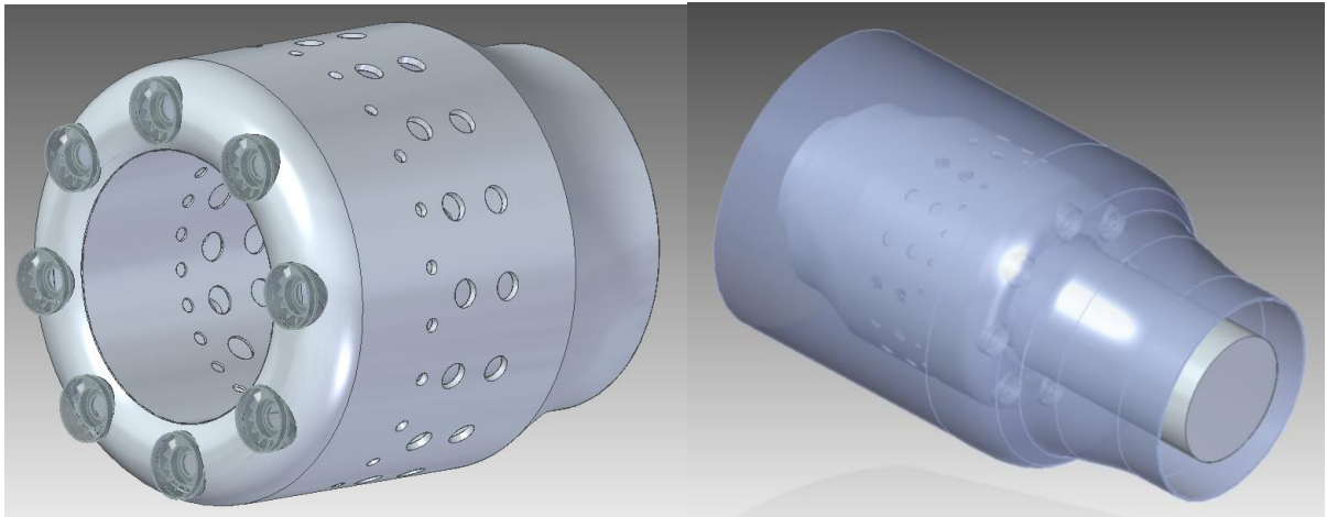
30. ábra: A tűzcső és a teljes égőtér modellje SolidEdge környezetben (saját kép)
