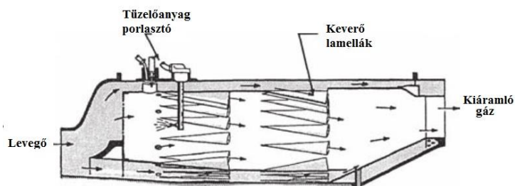
8. ábra: Metrowick hajtómű gyűrűs égőterének sematikus rajza [20]
