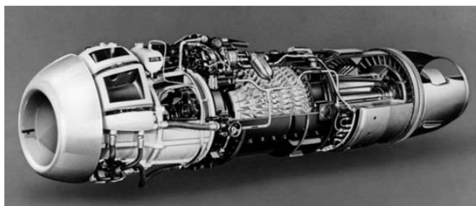
3. ábra: BMW 003 típusú hajtómű [11]
