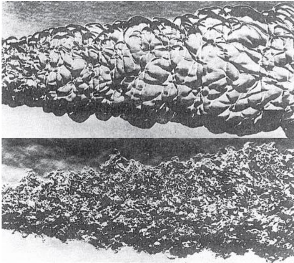
26. ábra: Sztöchiometrikus előkevert turbulens lángok (felül) u'=3,1 m/s, (alul) u'=30,5 m/s [25]
